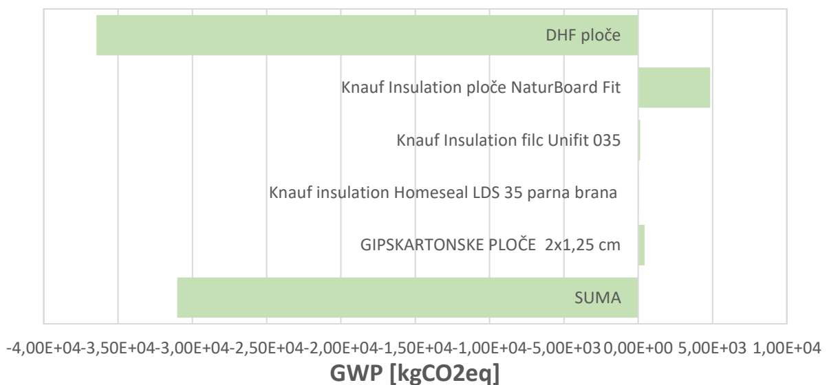
Graf 5.6 Međukatna konstrukcija – tavan: Ukupni modul A-C
