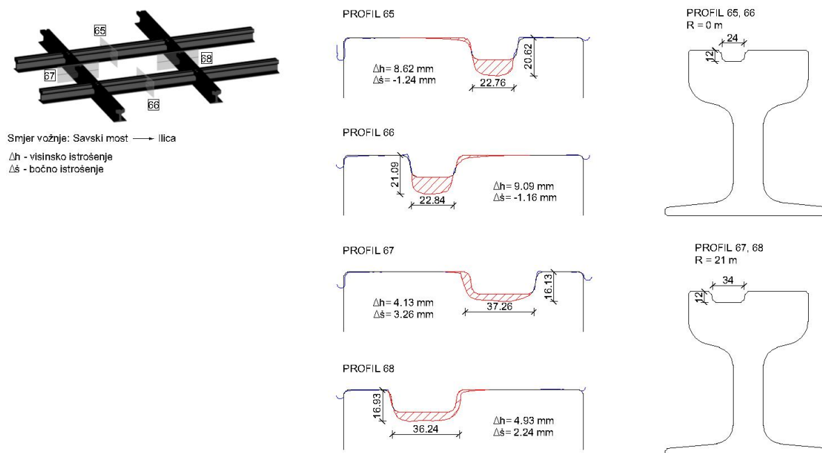
Slika 6. Grafička analiza istrošenja tračnica u križalištima
