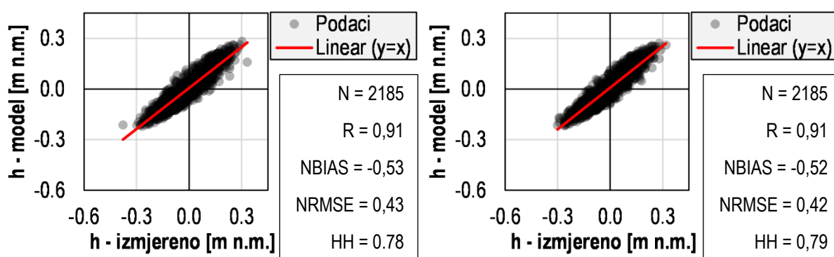
Slika 5-10 Dijagram raspršenja i statistički pokazatelji pouzdanosti modela koji daju uvid u odnos izmjerenih i modeliranih morskih razina na lokacijama ADCP-PL1 (lijevo) i ADCP-PL2 (desno) u LJETNOM razdoblju
