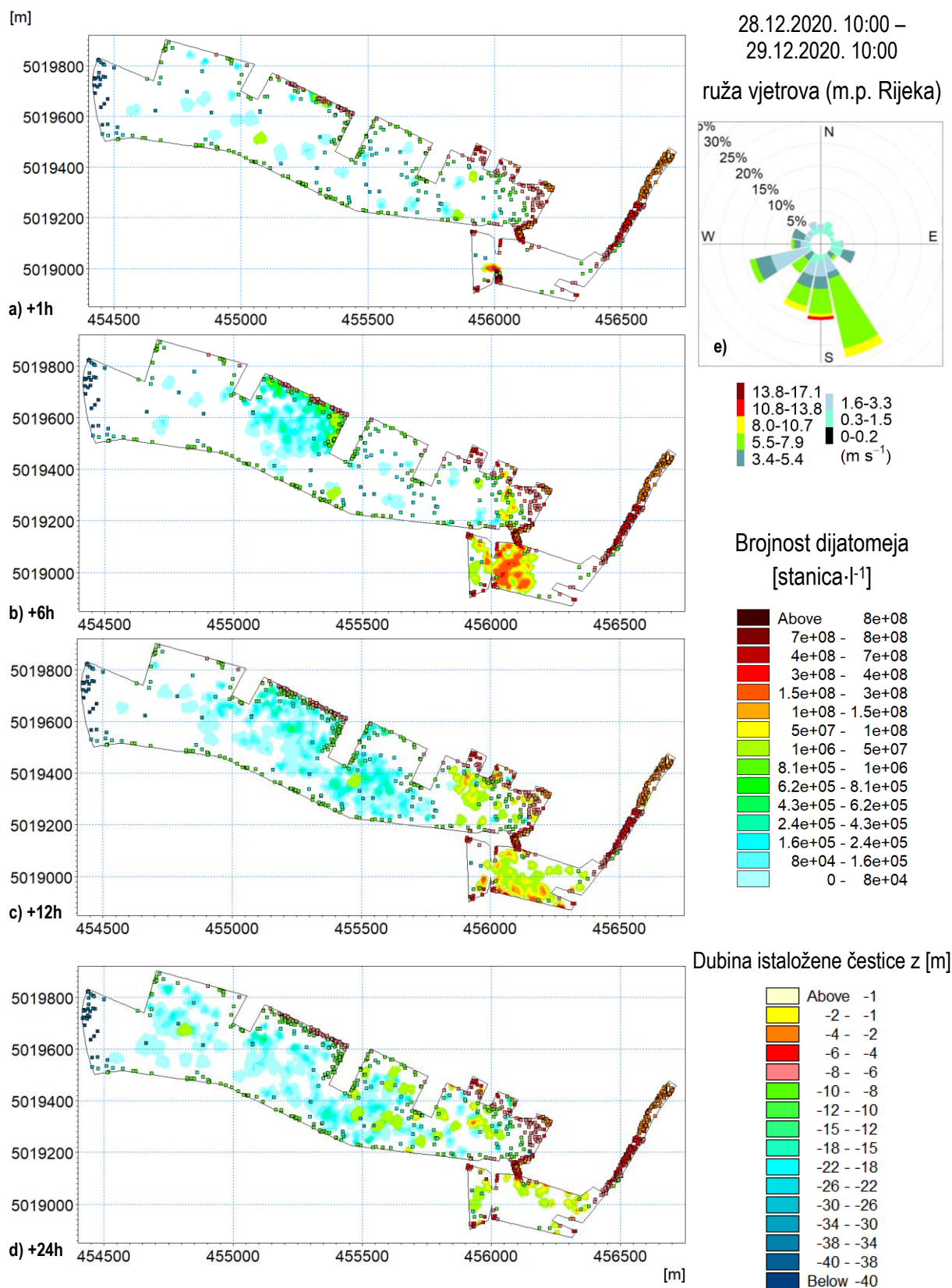
Slika 5-63 2D polja dijatomeja raspršenih u stupcu mora izražena u [stanica \cdot l ^{-1} ] s prikazom modelskih čestica istaloženih na dnu 1, 6, 12 i 24 [h] (a, b, c, d) nakon unosa modelskih čestica u trenutku 28.12.2020. 10:00, ruža vjetrova na m.p. Rijeka (e) u razdoblju od 28.12.2020. u 10:00 do 29.12.2020. u 10:00
