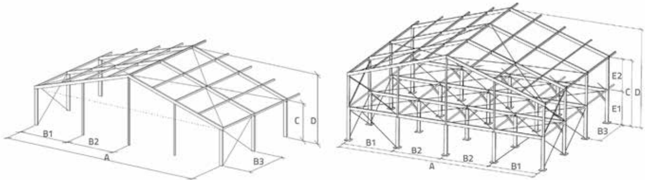
Slika 3. Okviri s ravnim prečkama P i P+1 - sa zategama i bez njih
