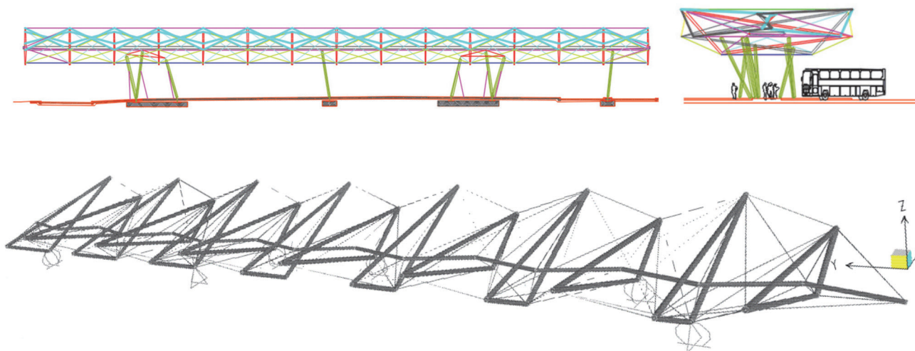
Slika 7. Idejno rješenje nadstrešnice Zračne luke u Čilipima (2005.)
