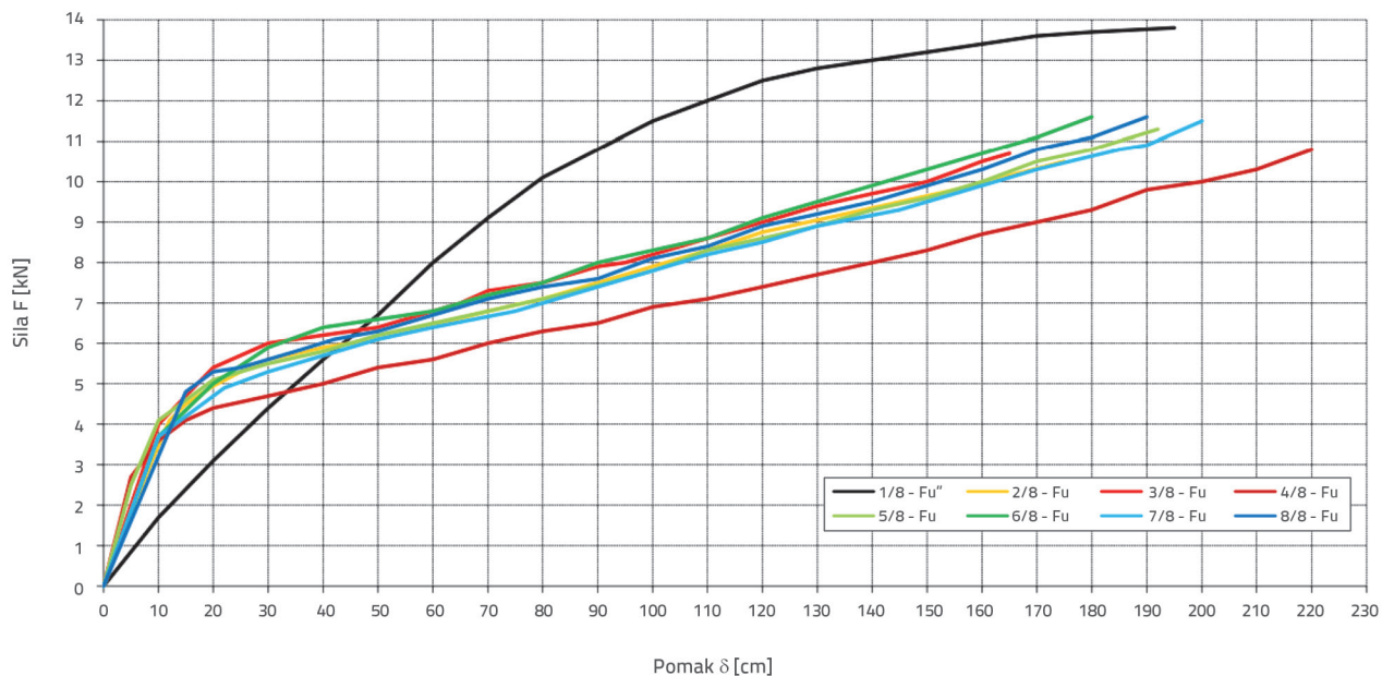
Slika 14. Preklapljeni dijagrami opterećenje – progib svih ispitanih uzoraka stupova (dijagram konvencionalno armiranog stupa istaknut je crnom bojom)
