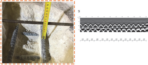
Slika 8. Određivanje rasporeda armature monolitne armiranobetske ploče
