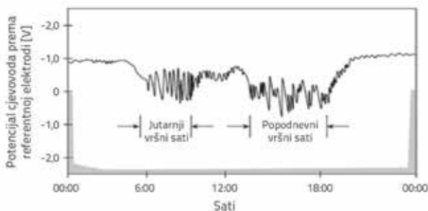
Slika 8. Potencijal cjevovoda mjeren u periodu od jednog dana [29]
