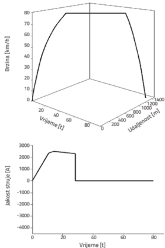
Slika 5. Dijagram ovisnosti vremena, brzine i prijeđene udaljenosti prilikom kretanja tračničkog vozila (gore), jakost struje potrebne vozilu s obzirom na različite načine kretanja (dolje), prema [17]
