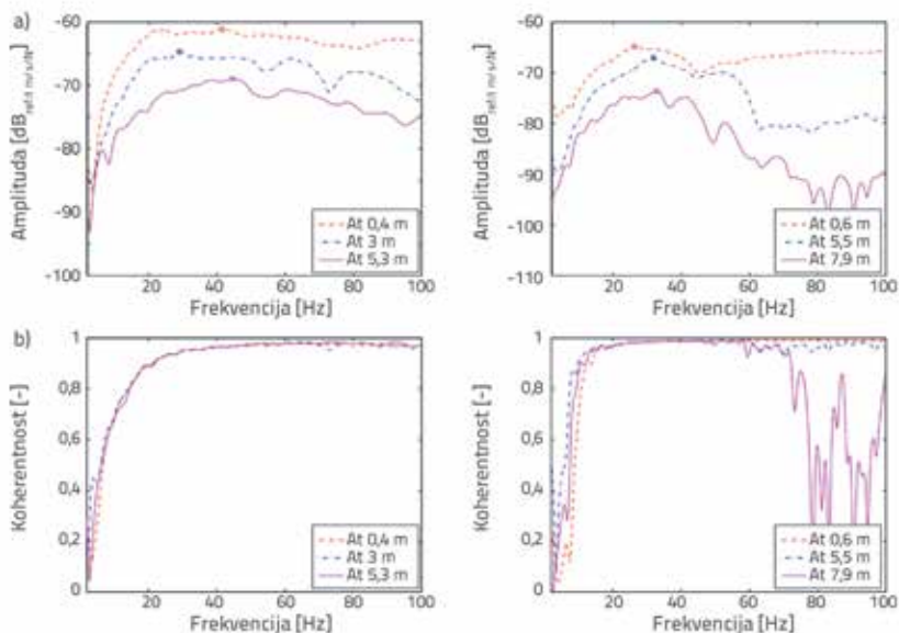
Slika 10. Funkcije mobilnosti prenosa, frekvencija i koherentnost: a) kolosijek sa zastornom prizmom, b) kolosijek na čvrstoj podlozi [26]
