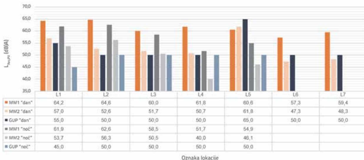
Slika 20. Ekvivalentne razine buke svih vozila koja su prošla pored mjernih mjesta MM1 i MM2
