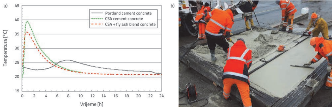
Slika 4. a) Usporedba prirasta temperature portlandcementnog betona, betona sa CSA cementom te betona sa CSA cementom i letećim pepelom tijekom 24 sata [37]; b) Betoniranje betonom pripremljenim sa CSA cementom na uzletno-sletnoj stazi (slika: T. Conjar, TPA)
