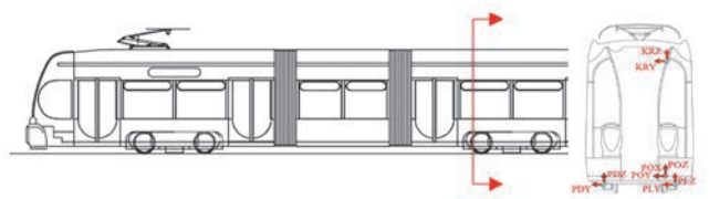
Slika 7. TMK 2200 (Končar KEV) tramvaj i pozicije akcelerometara za ispitnu dionicu 2
