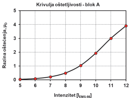
Slika 4. Krivulja oštećljivosti
