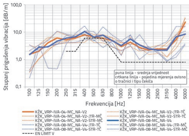
Slika 22. Usporedba stupnja prigušenja vibracija u vertikalnom smjeru na dvije pozicije akcelerometara (V2 i V4)
