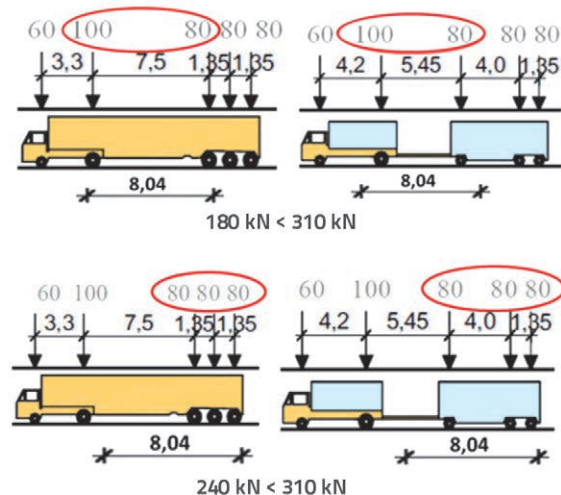
Slika 6. Utjecaj osovinskog razmaka najtežih osovina reprezentativnih vozila tipa 5 (tegljač) i 6 (teretni kamion s prikolicom) pri djelovanju na most raspona manjeg od ukupne duljine vozila
