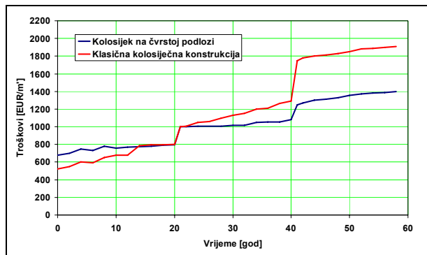
Slika 4. Usporedba troškova klasičnog kolosijeka i kolosijeka na čvrstoj podlozi, [5]
