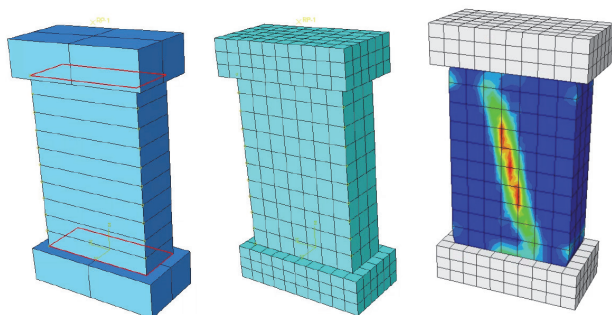
Slika 8. Zid obrađen za primjer. Označeni setovi/mesh/rezultati
