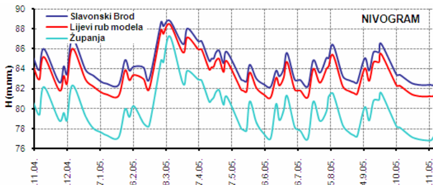
Slika 5. Nivogram Save na postajama Slavonski Brod i Županja tijekom razdoblja 28.11.04. do 28.11.05. i usvojeni nivogram Save na lokaciji lijevog ruba modeliranog područja
