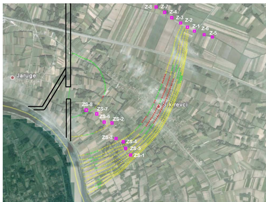
Slika 13. Napredovanje tvari iz Save prema zdencima crpilišta u Sikirevcima i Gundincima
