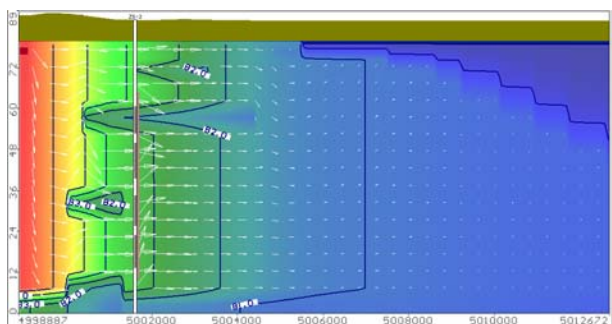
Slika 10. Ekvipotencijale i vektori brzina u vertikalnoj YZ ravni modela koje prolaze kroz zdenac ZS-2 u Sikirevcima za visoke vode rijeke Save za maksimalnu projektom predviđenu izdašnost crpilišta Sikirevci od Q_{SIK} = 1000 l/s i maksimalnu izdašnost crpilišta Gundinci Q_{GUN} = 1000 l/s
