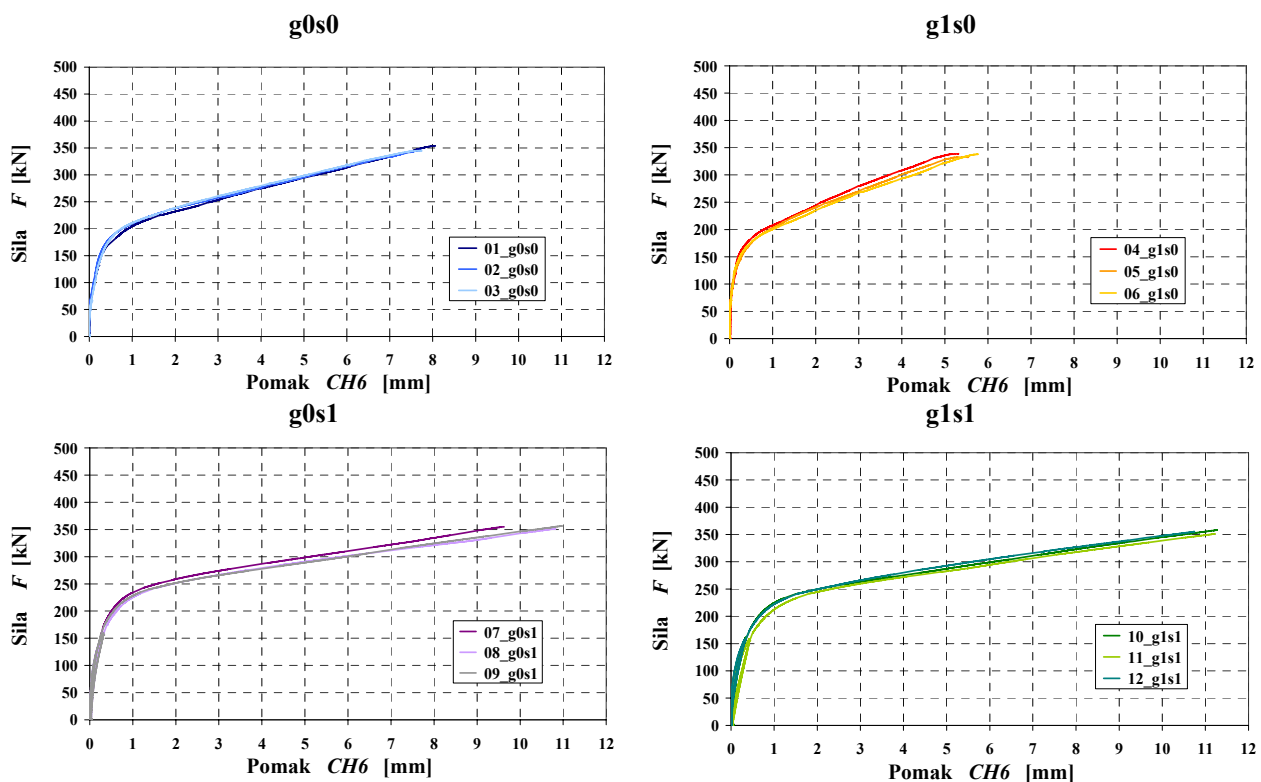
Slika 11. Odizanje kutnika u osi vijaka 80 mm od ruba, kanal CH 6
