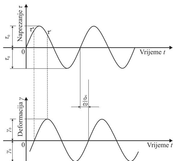
Slika 6. Dijagrami posmičnih napreznja i deformacija u ovisnosti o vremenu [3]
