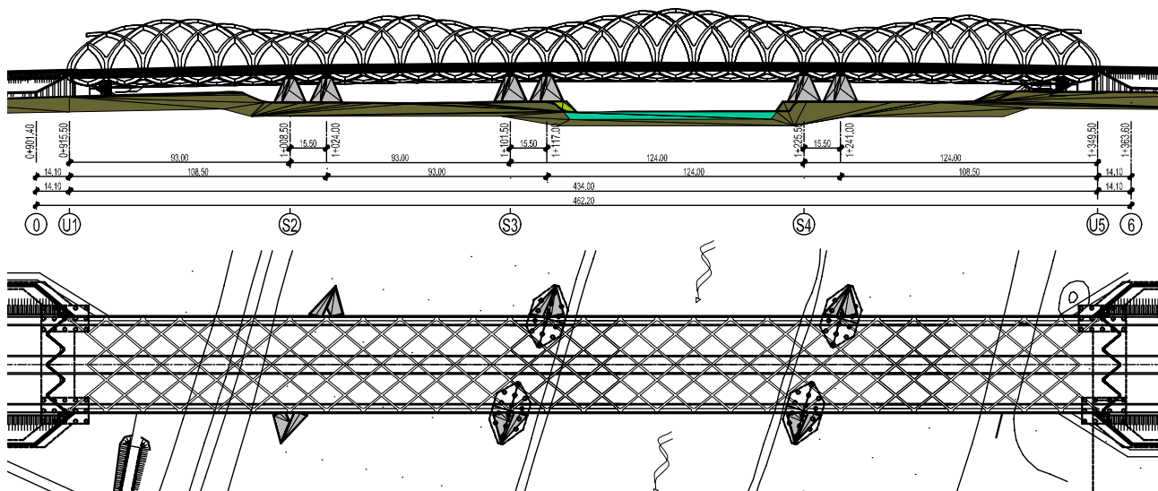
Slika 3. Uzdužni presjek i tlocrt mosta Bundek
