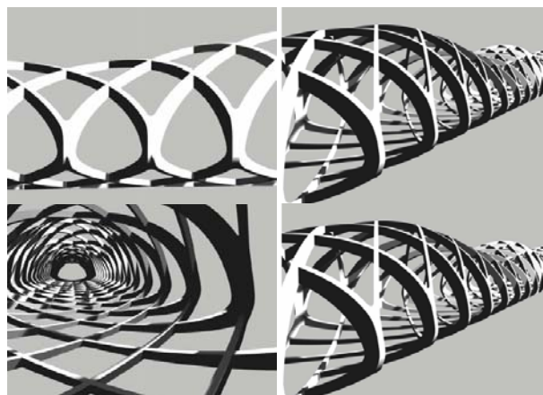
Slika 5. Pravilna struktura konstrukcije mosta Bundek
