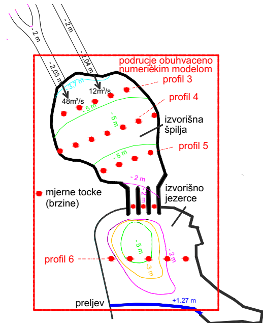
Slika 3. Dubine na području izvorišne špilje, izvorišnog jezera i prelivnog praga i položaji mjernih točaka na kojima su mjerene brzine na fizikalnom modelu
