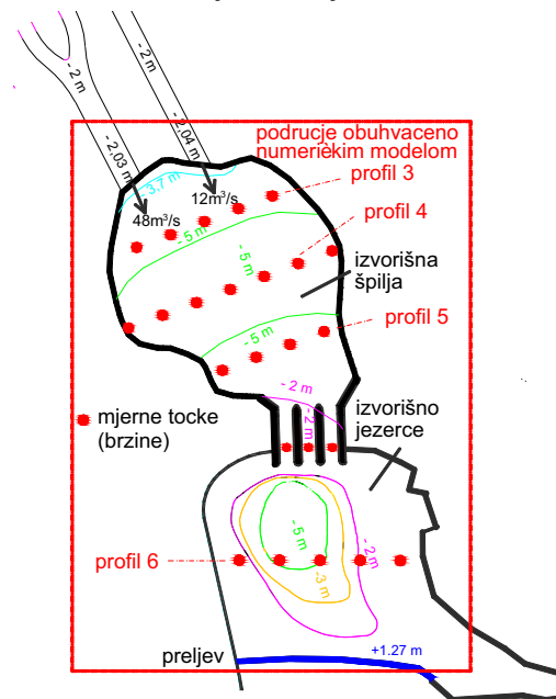
Slika 3. Dubine na području izvorišne špilje, izvorišnog jezera i preljevnog praga i položaji mjernih točaka na kojima su mjerene brzine na fizikalnom modelu
