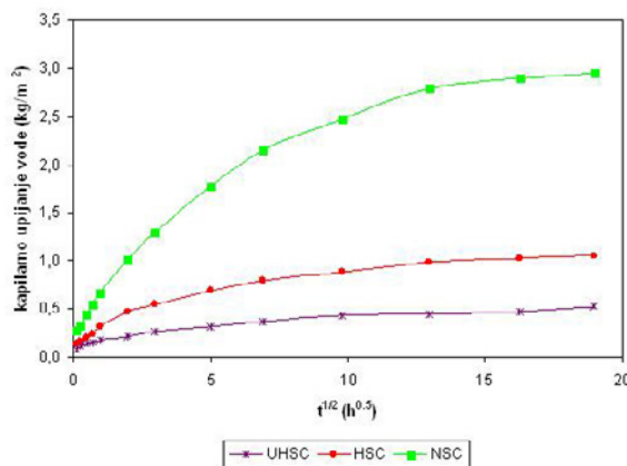
Slika 8. Dijagrami srednjih vrijednosti ispitivanja kapilarnog upijanja vode
