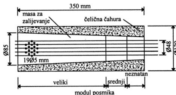
Slika 4. Primjer sidrenja CFRP kabela s prikazom promjene modula posmika mase za zalijeвање čahure [11, 21]
