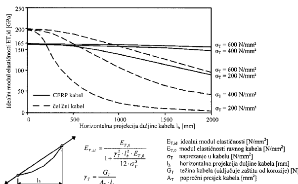
Slika 1. Idealni modul elastičnosti E_{T, id} vješaljka (zatega) od čelika ili CFRP-a ovisno o horizontalnom rasponu zatege [20]
