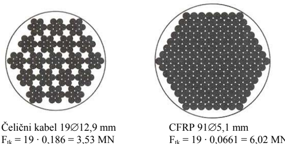
Slika 8. Presjeci užadi ovješnog mosta Dintelhaven [20]
