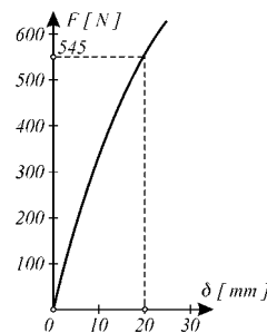
Slika 11. Dijagram bočnih pomaka Z- profila
