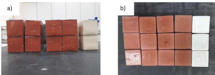
Slika 3. Sintetizirani geopolimerni uzorci; sdesna nalijevo referentni uzorak (bijeli) te 20 mas.% zamjena metakaolina s boksitnim ostatkom (nekalcinirani - RT, 500^\circ\text{C} , 600^\circ\text{C} , 700^\circ\text{C} )
