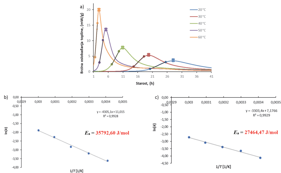
Slika 1. Rezultati mjerenja izoternnom kalorimetrijom i grafički prikaz linearanog dijela krivulja (a); Određivanje E_a u ovisnosti o najvećoj brzini hidratacije, \ln(k) , o 1/T (b); Određivanje E_a ovisno o prosječnoj brzini hidratacije, \ln(k) , o 1/T (c)
