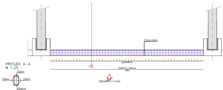
Slika 22 Plan armature temeljne vezne grede
