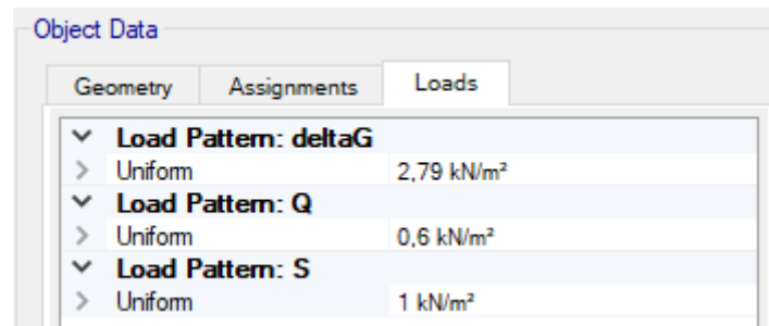
Slika 54. Opterećenje prema Eurokodu
