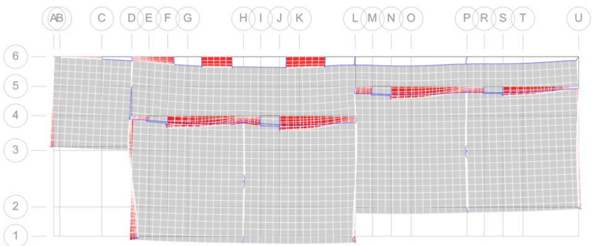
Slika 40: Sedmi oblik titranja u kojem se aktivira 75% mase u y smjeru - 2D
