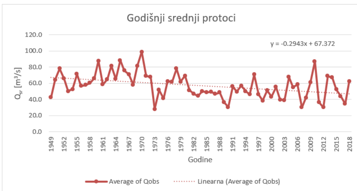
Slika 22: Niz srednjih godišnjih protoka Cetine na mjernoj postaji Han u razdoblju od 1949. do 2018. godine
