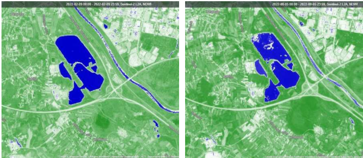
Slika 5. Usporedba vodostaja jezera Rakitje za različite periode; Lijevo - 9. veljače 2022., Desno – 5. kolovoza 2022.
