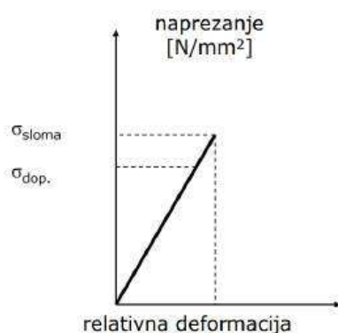
Slika 4: Radni dijagram stakla (Izvor: [3])
