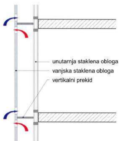
Slika 36: Ventilirana prekinuta obloga (Izvor: [46])
