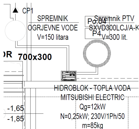
Slika 22.: Komponente sustava za pripremu sanitarne tople vode (Izvor: [25])
