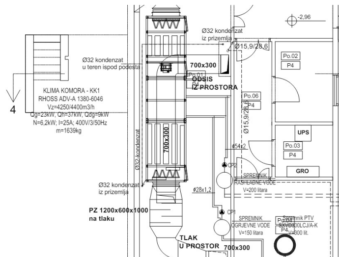
Slika 21.: Različite komponente sustava klimatizacije koje zajedno osiguravaju kontrolu temperature i kvalitete zraka unutar zgrade (Izvor: [25])
