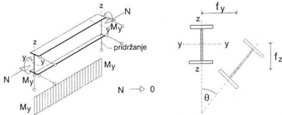
Slika 9.: Bočno-torzijsko izvijanje [2]
