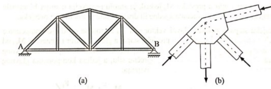
Slika 7. Detalj vezivanja štapova [3]
