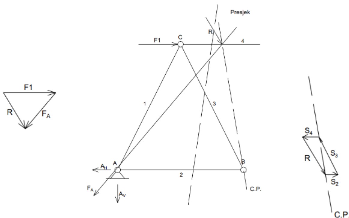
Slika 30. Određivanje sila u štapovima rešetkastog nosača Culmannovom metodom [10]
