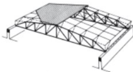
Slika 16. Krovni nosači [5]
