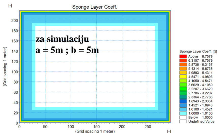
Slika 2.2 Primjer „sponge layera“ za apsorpciju valne energije i onemogućenje valne refleksije od rubova modela (razmaci između konvertera a = 5\text{m} i b = 5\text{m} , vidi tablicu 2.1)
