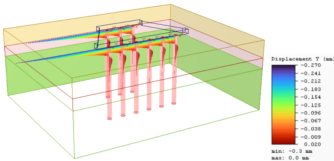
Slika 47.: Poprečni pomaci u y -smjeru za GSN
