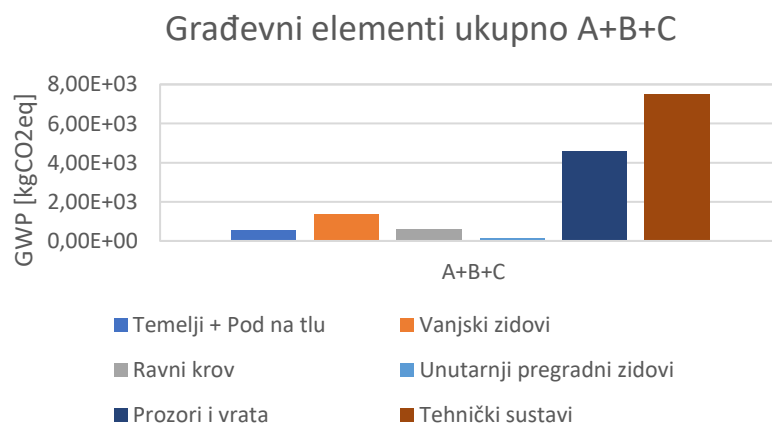
Slika 22. Potencijal globalnog zatopljenja ugrađenih građevnih elemenata od faze A do faze C- mobilna kućica 3
