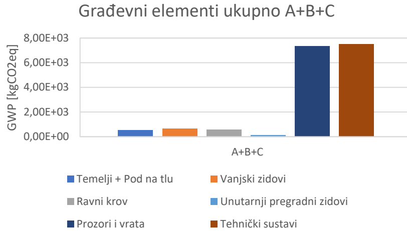
Slika 20. Potencijal globalnog zatopljenja ugrađenih građevnih elemenata od faze A do faze C- mobilna kućica 1
