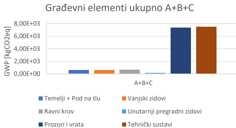
Slika 21. Potencijal globalnog zatopljenja ugrađenih građevnih elemenata od faze A do faze C- mobilna kućica 2
