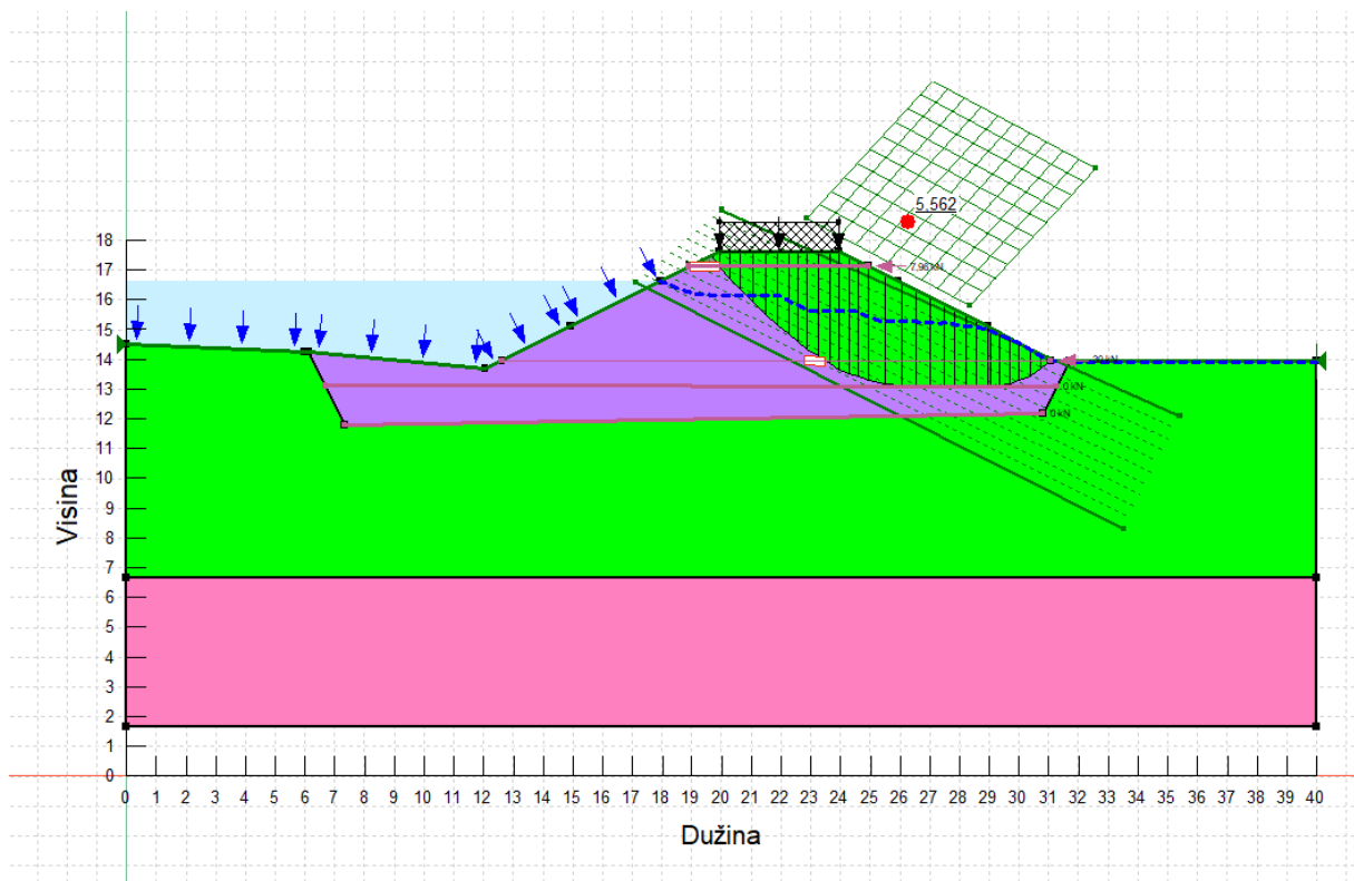
Slika 54. Stabilnost desnog pokosa pri uvjetima visoke vode, negativnim vertikalnim koeficijentom ubrzanja i u nedreniranim uvjetima
