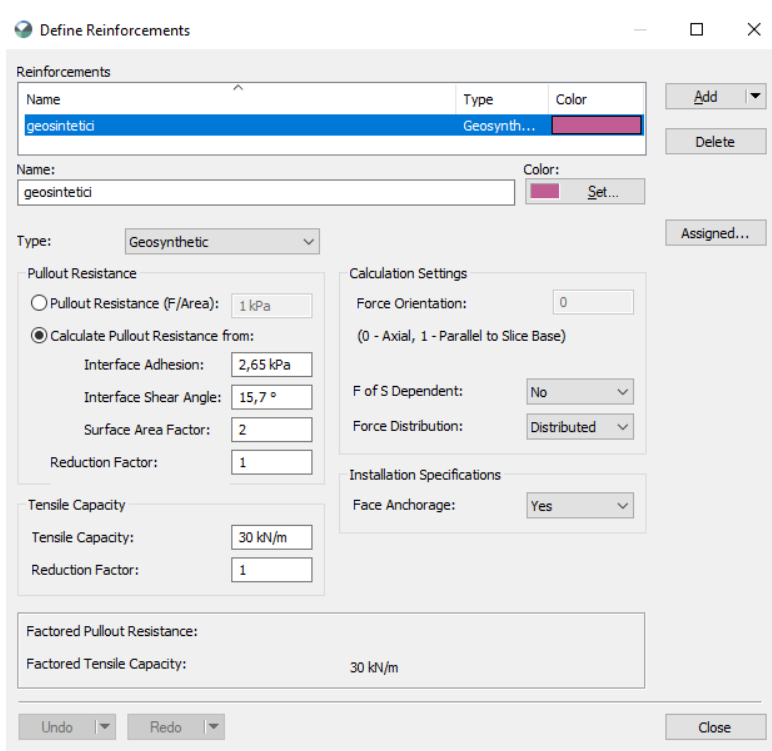
Slika 41. Karakteristike geomreža
