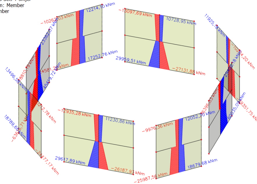
Slika 96.: Moment savijanja u ravnini (Seizmička kombinacija Y) - zid 6b
