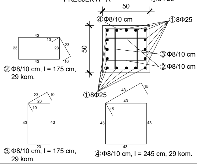
PRESJEK A - A
