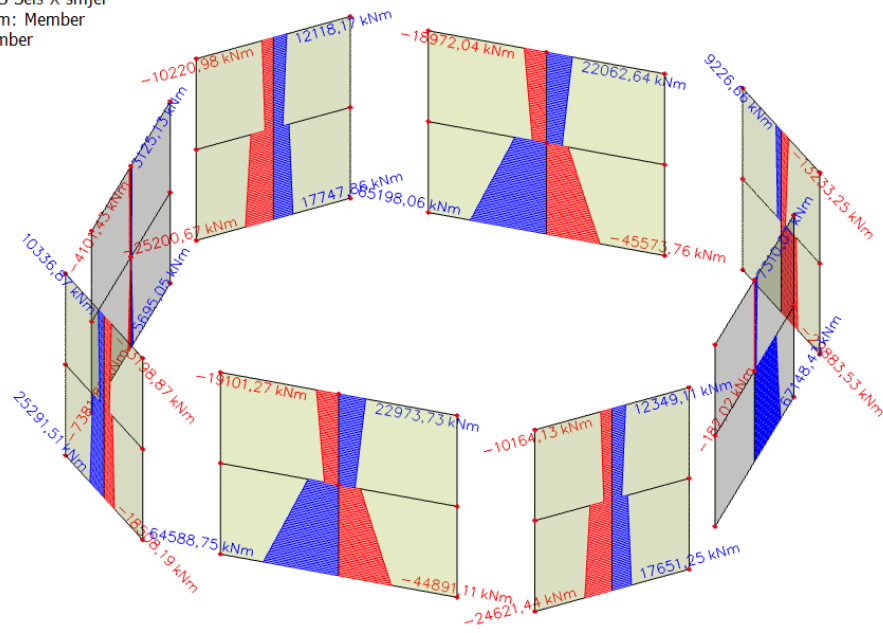
Slika 95.: Moment savijanja u ravnini (Seizmička kombinacija X) - zid 6a
