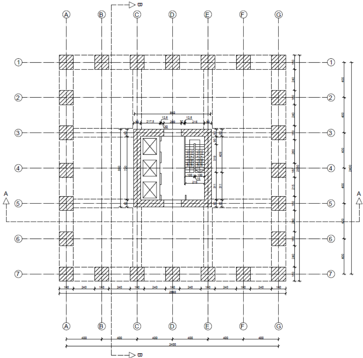
Slika 1. Tlocrt etaža 1-14
