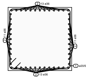
Presjek 1 - 1
