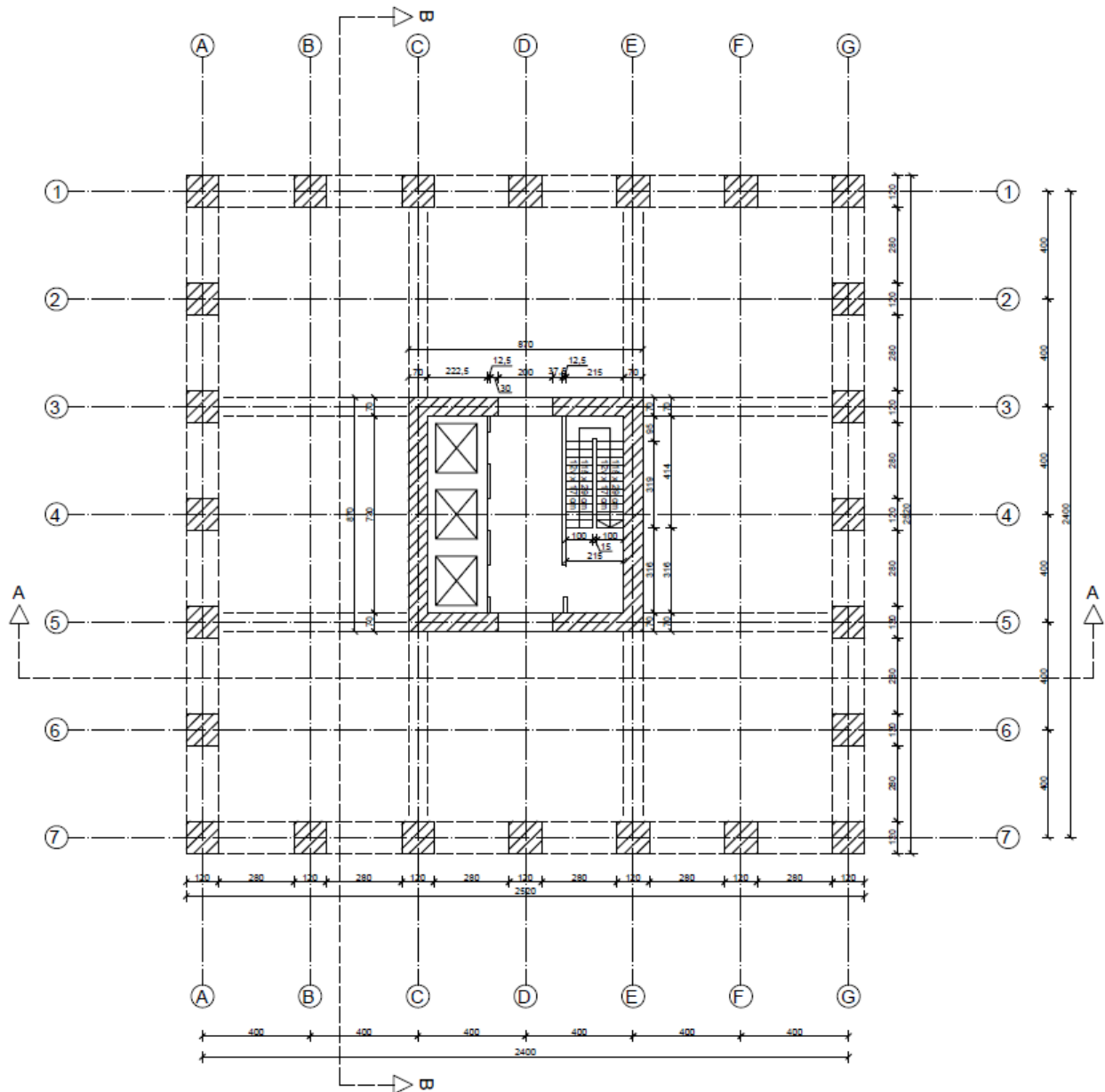
Slika 7. Tlocrt etaža 37-50
