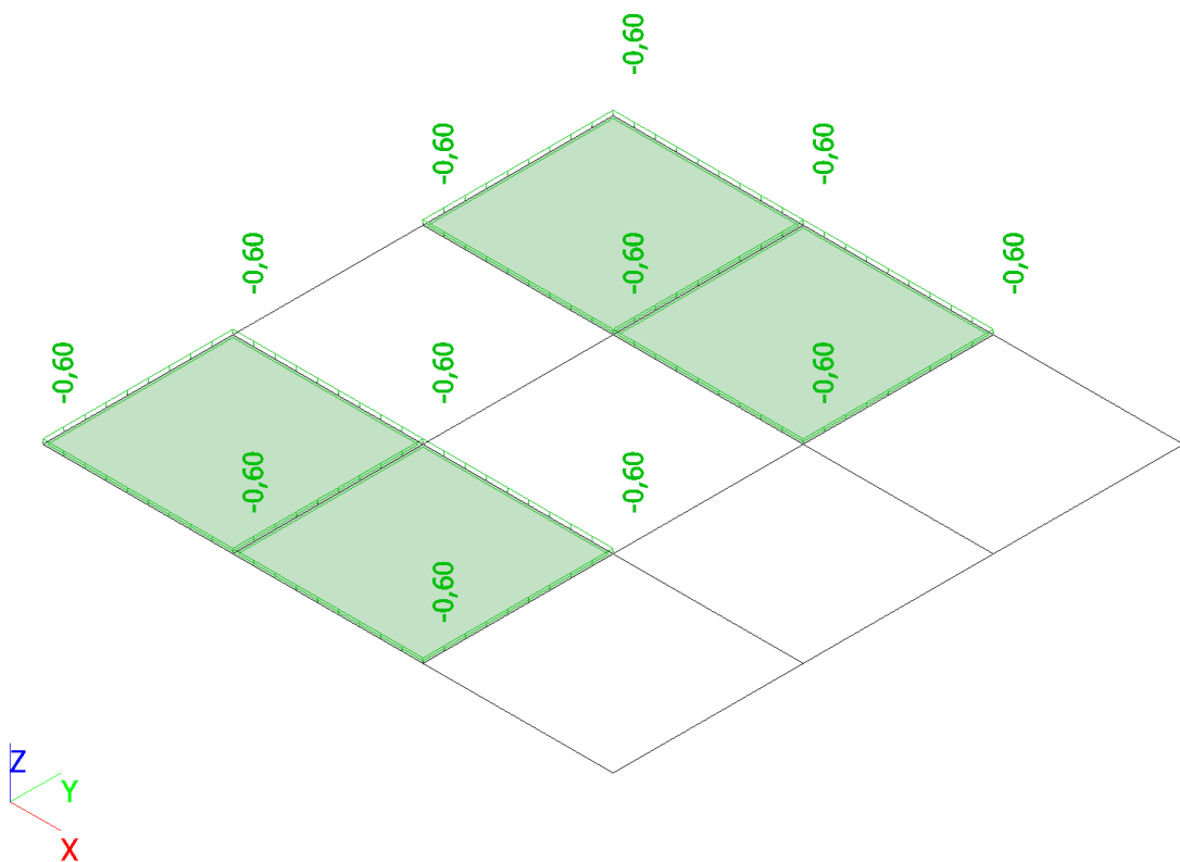
Slika 42. Uporabno opterećenje krovne konstrukcije [ \text{kN/m}^2 ]
