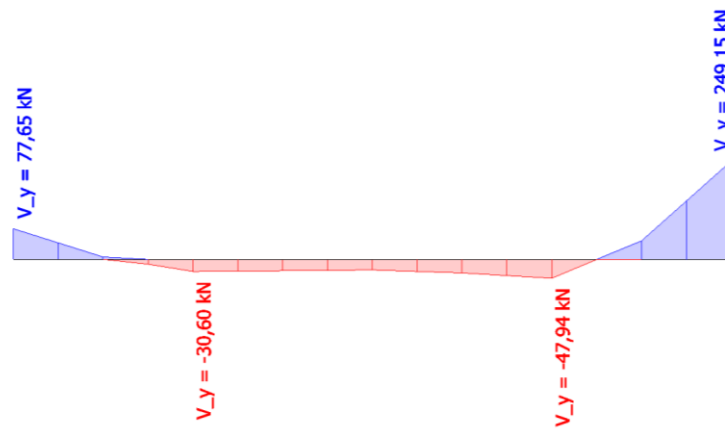
Slika 171. Grafički prikaz mjerodavne poprečne sile za grede 160/150 cm (nazovistalna kombinacija)
