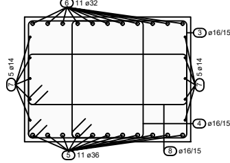
Presjek 2 - 2
