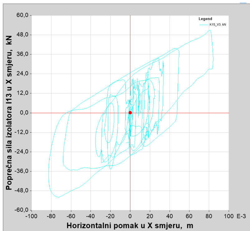
Slika 64.: Horizontalna sila i pomak u smjeru X izolatora I13 [10]
