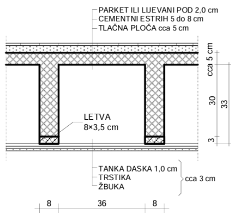
AB SITNOREBRATA STROPNA KONSTRUKCIJA
