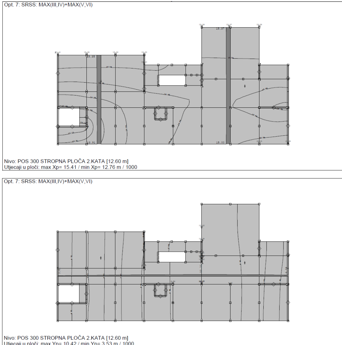
Slika 81.: Pomaci ojačane konstrukcije [3]
