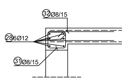
PRESJEK 23-23 M=1:25
