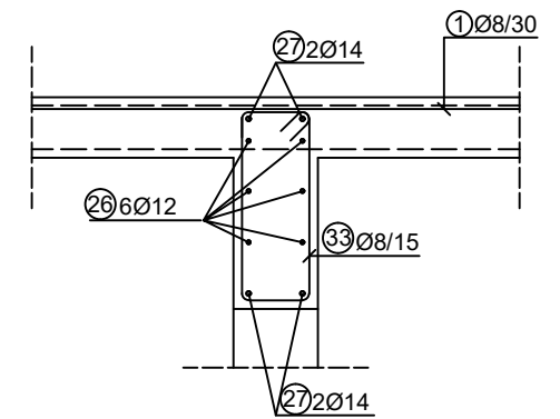
PRESJEK 20-20 M=1:25
