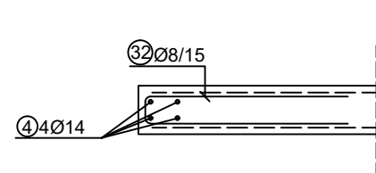
PRESJEK 22-22 M=1:25
