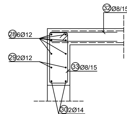
PRESJEK 24-24 M=1:25
