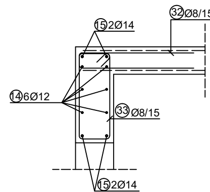
PRESJEK 6-6 M=1:25
