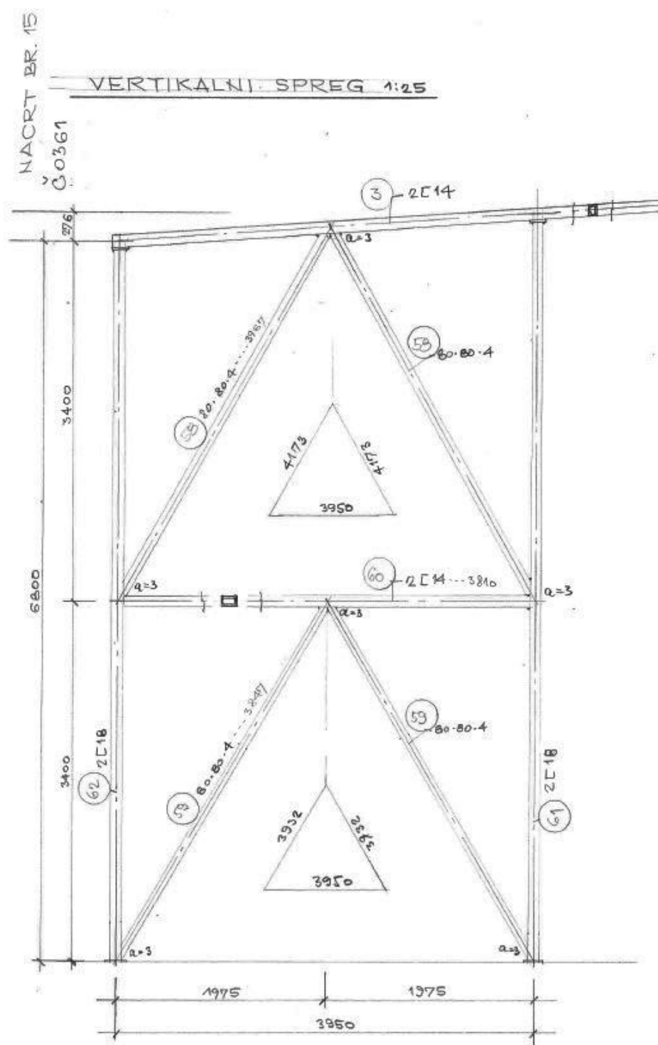
Slika 33. Vertikalni spreg
