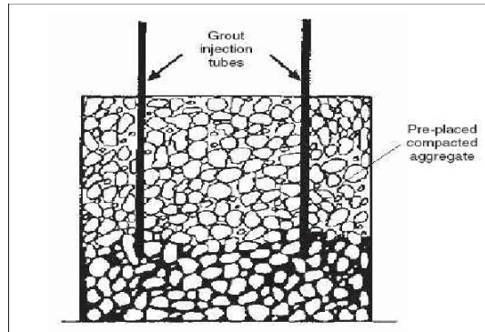
Slika 13 Colcrete sistem
