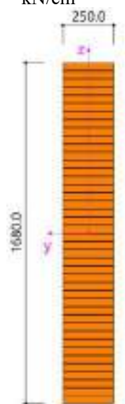
Slika 4.1 Poprečni presjek glavnog nosača [mm]
