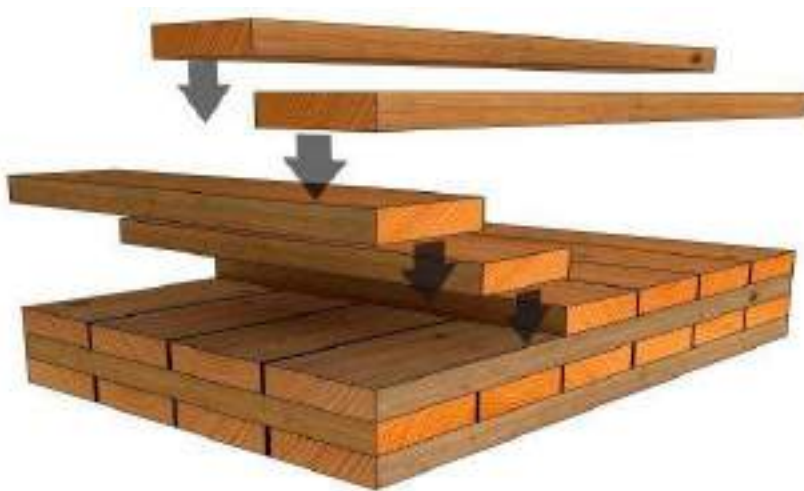
Slika 1.5 Raspored slojeva u križno lameliranom drvu [14]
