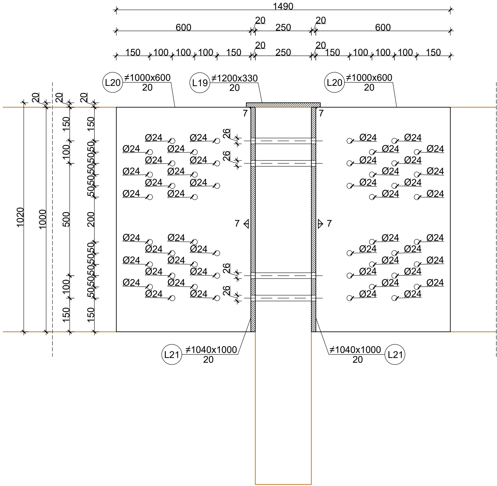
Detalj 6 - detalj spoja sekundarnog i glavnog nosača M 1:10
