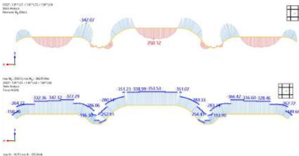
Slika 4.18 Dijagram momenata savijanja M_y [kNm] i uzdužnih sila N [kN] – najveći moment savijanja
