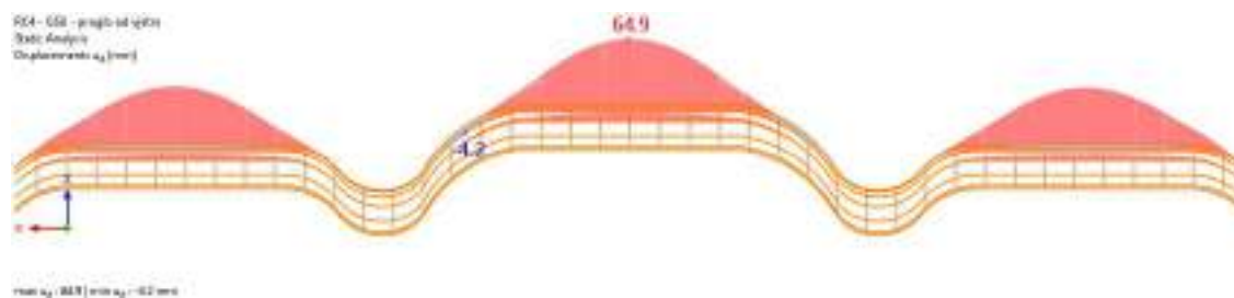
Slika 5.5 Anvelopa progiba uslijed opterećenja vjetra
