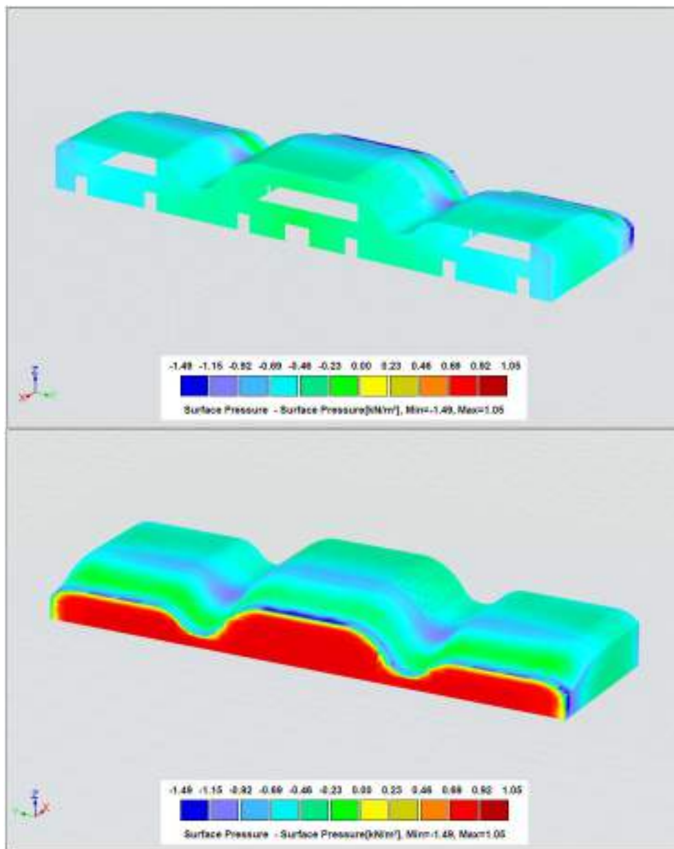
Slika 3.15 Opterećenje vjetra za slučaj 10 u \text{kN/m}^2
