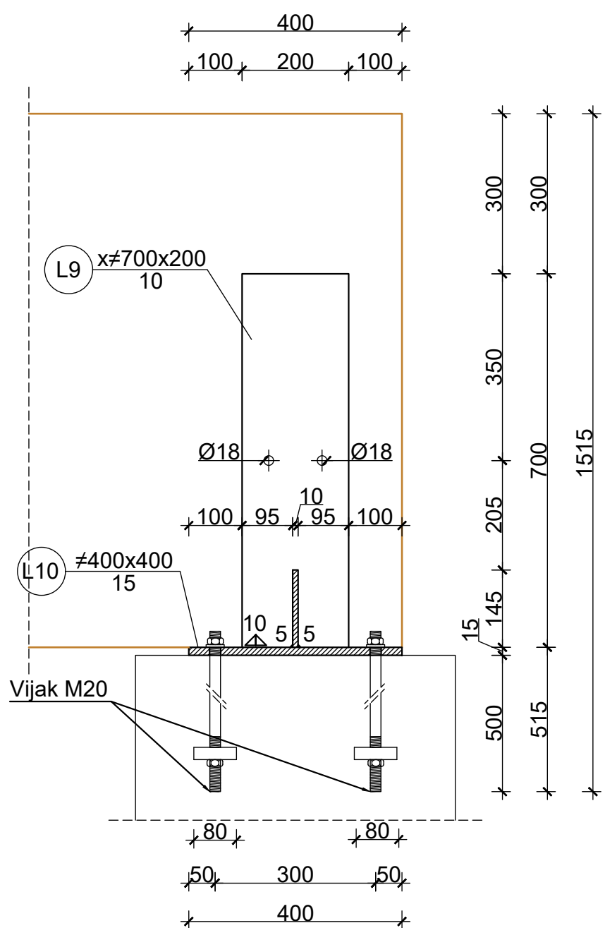
Detalj 3 - detalj nepomičnog ležaja sekundarnog nosača M 1:10
