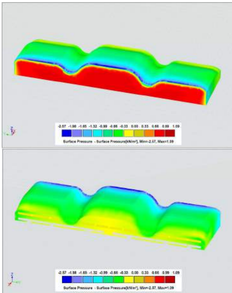
Slika 3.11 Opterećenje vjetra za slučaj 6 u \text{kN/m}^2
