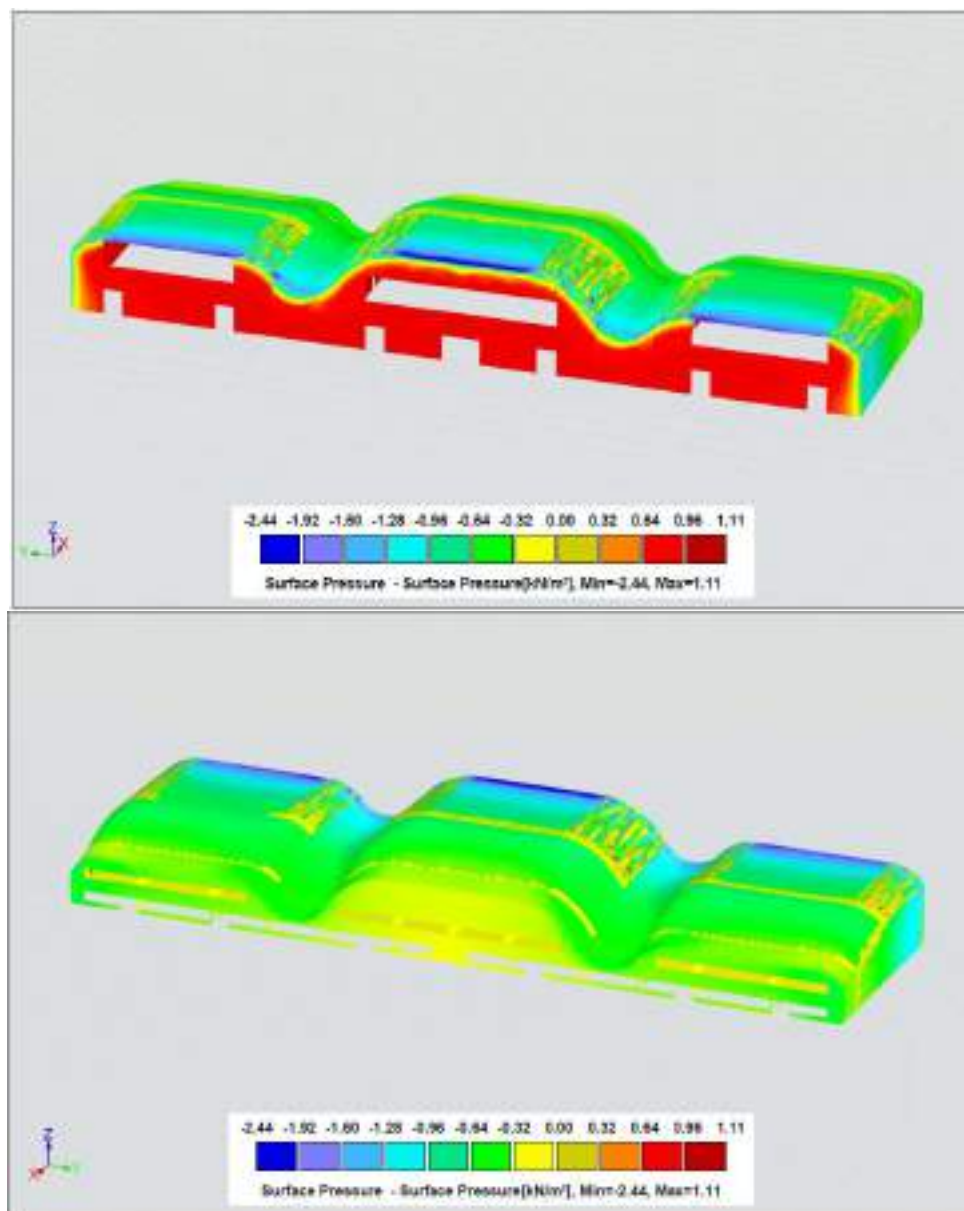
Slika 3.10 Opterećenje vjetra za slučaj 5 u \text{kN/m}^2
