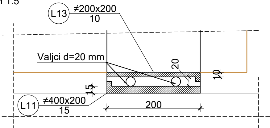
Presjek kroz ležaj M 1:5
