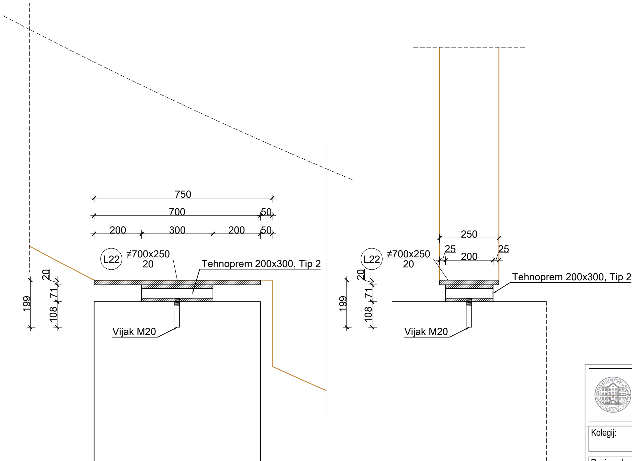
Detalj 7 - detalj oslanjanja glavnog nosača na zid M 1:10
