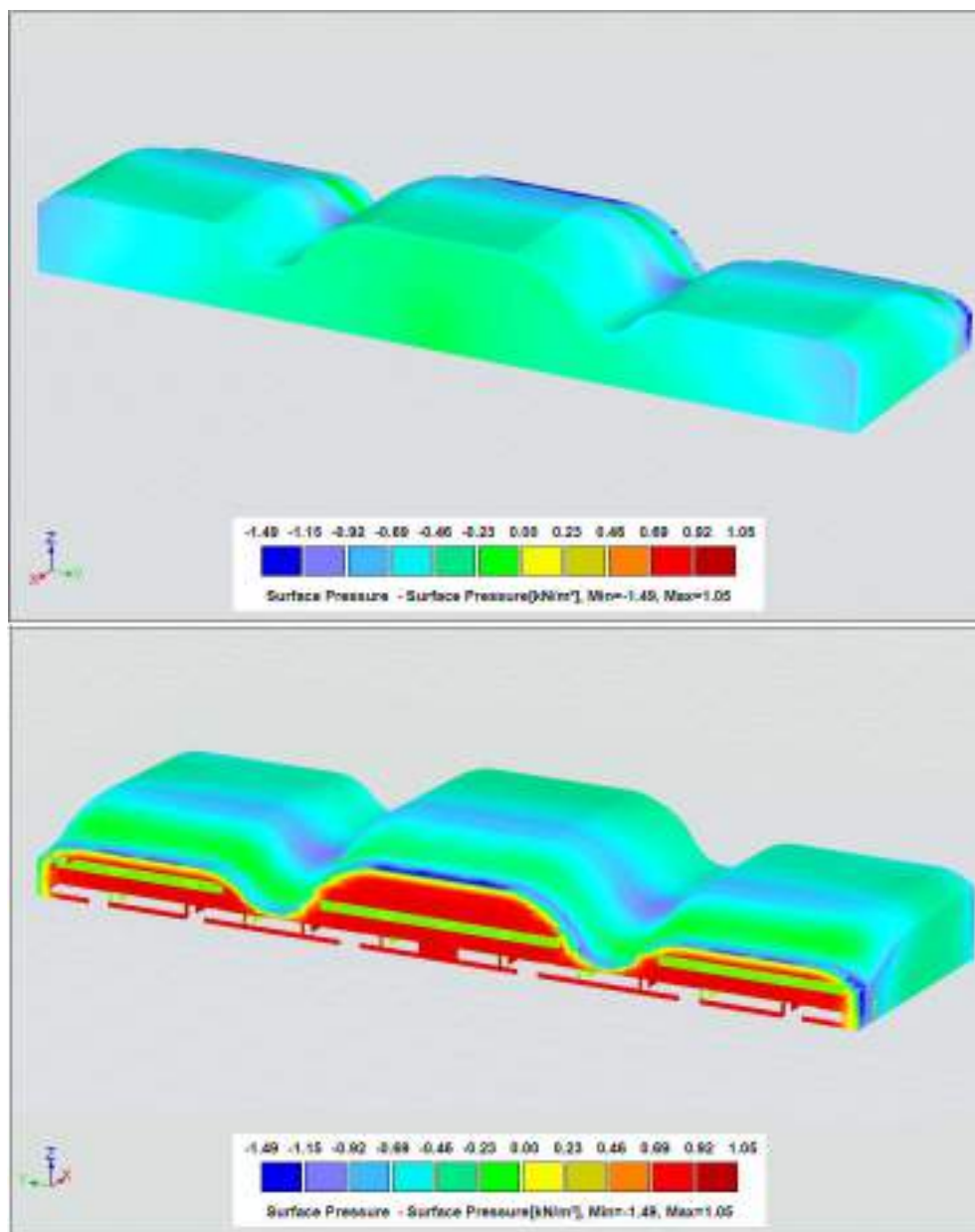
Slika 3.17 Opterećenje vjetra za slučaj 12 u \text{kN/m}^2
