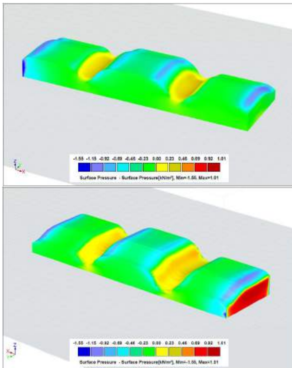
Slika 3.12 Opterećenje vjetra za slučaj 7 u \text{kN/m}^2
