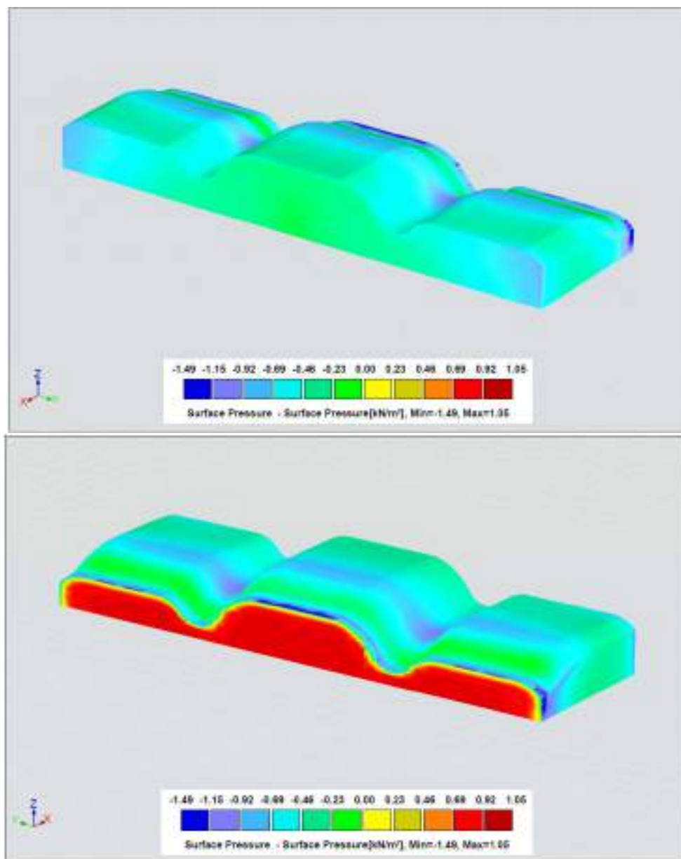
Slika 3.14 Opterećenje vjetra za slučaj 9 u \text{kN/m}^2
