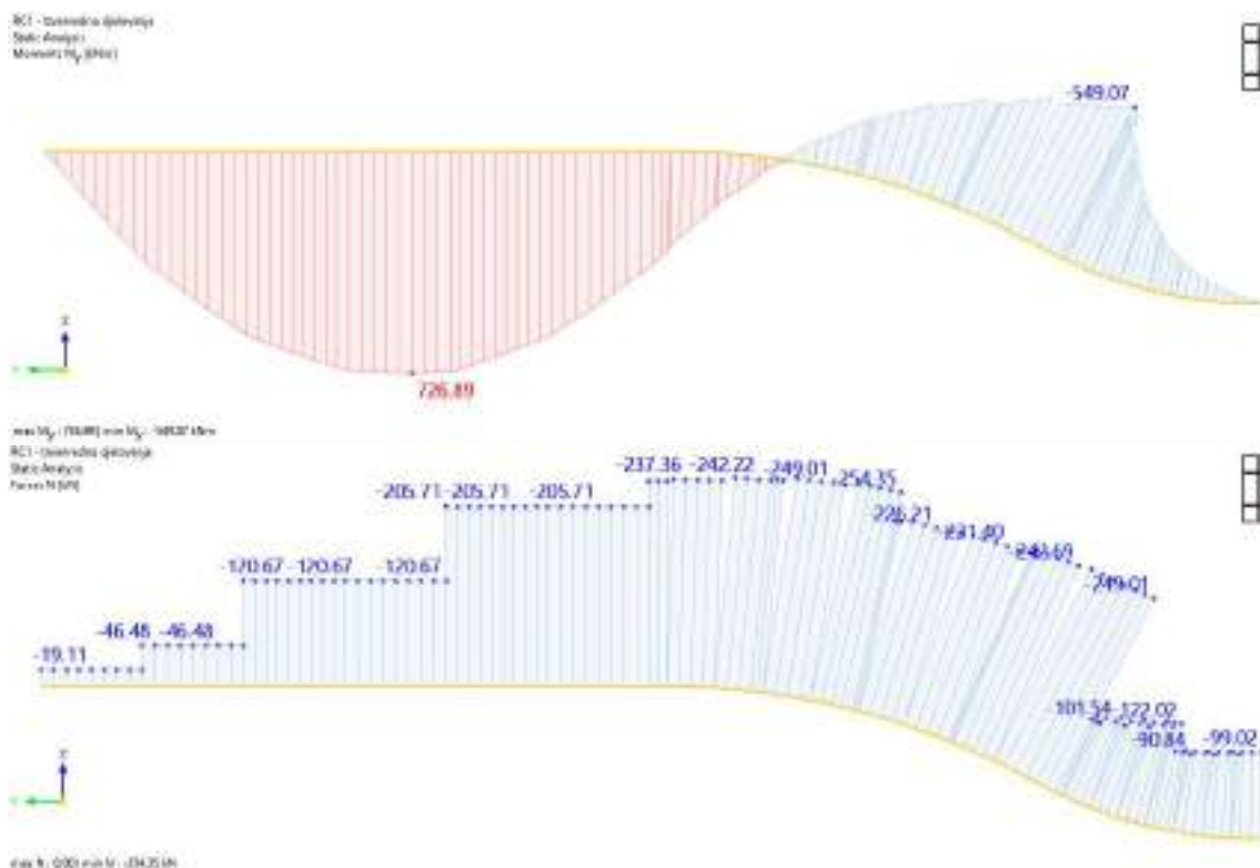
Slika 6.7 Dijagram momenata savijanja M_z [kNm] i uzdužnih sila [kN] za slučaj najvećeg momenta savijanja
