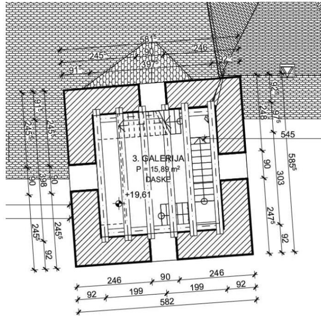
Slika 19. Pravilan tlocrt zvonika na višim etažama (Foretić i Trogrlić, 2021)
