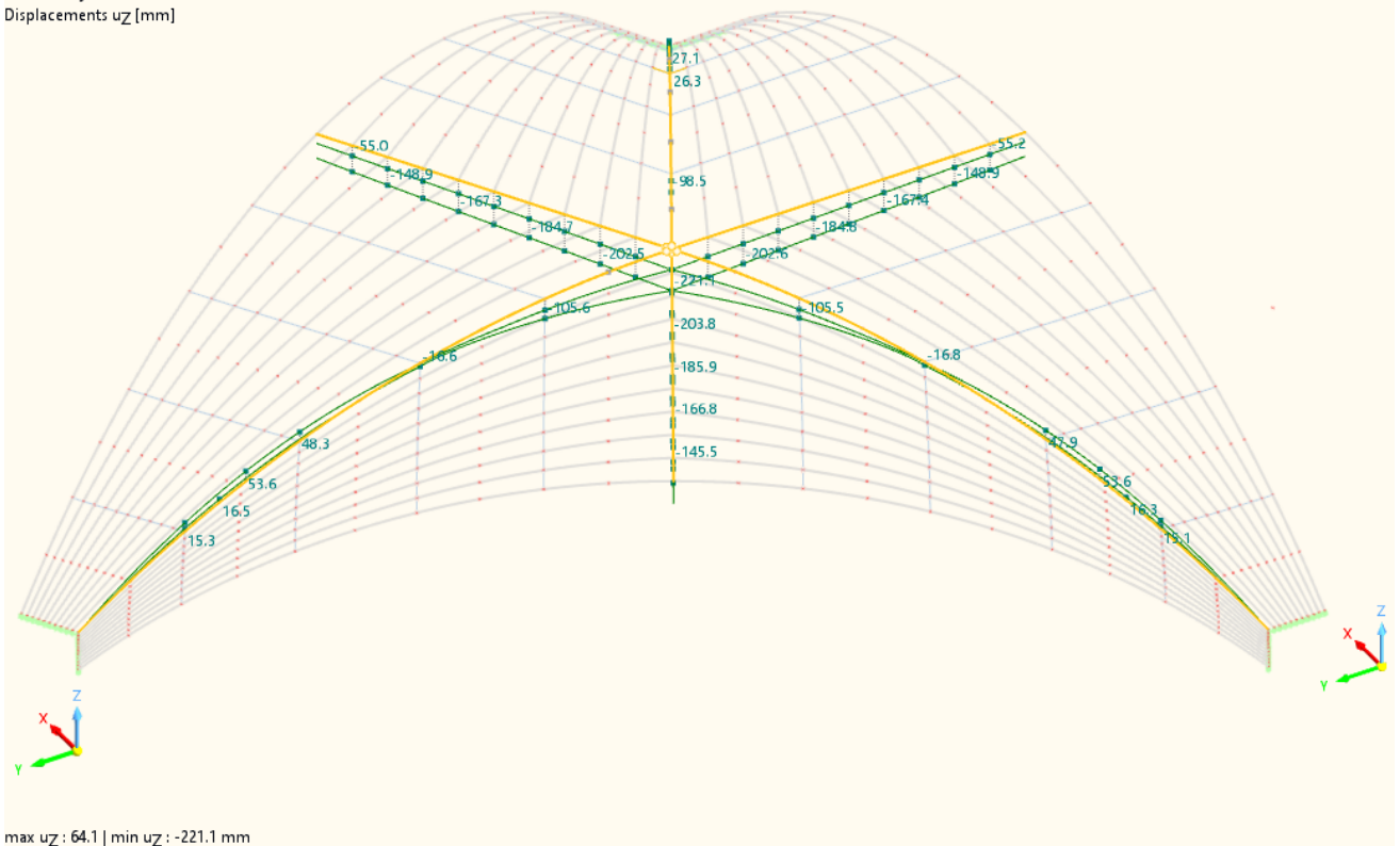
Slika 41. RC4 – Pomaci u_z – max vrijednost
