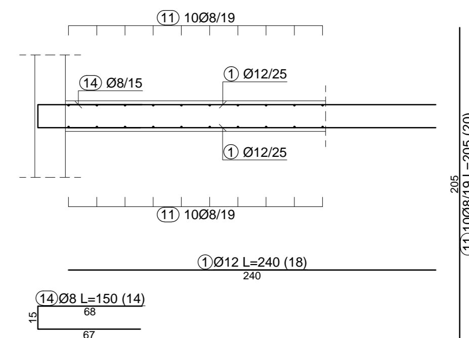
PRESJEK 3-3 MJ 1:25
