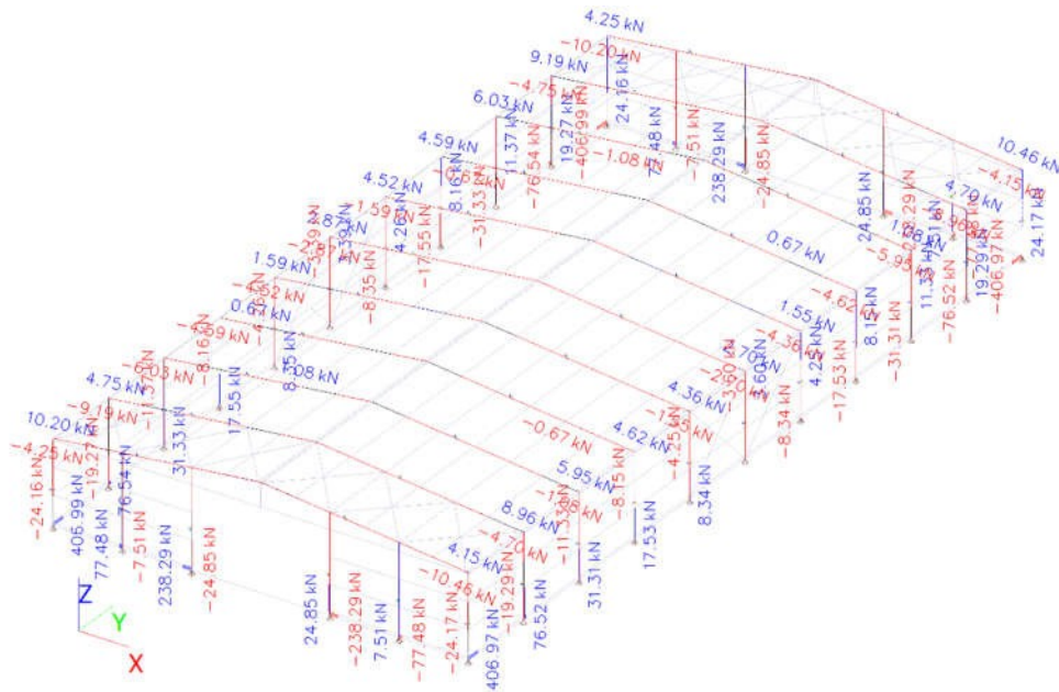
Slika 54. Rezne sile – poprečna sila
