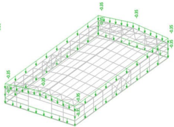
Slika 29.LC3 – dodatno stalno - zidovi
