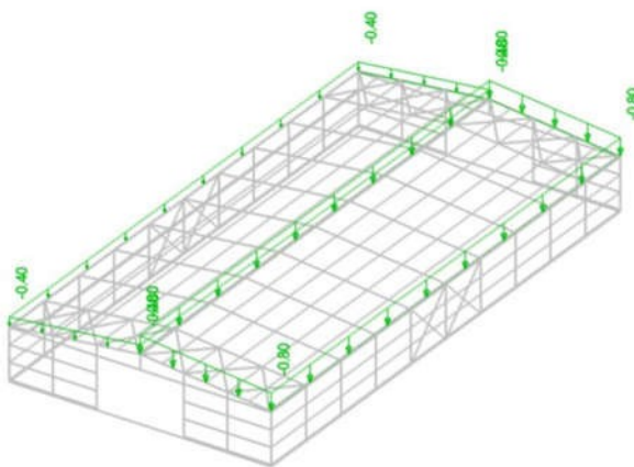
Slika 32.LC6 – snijeg desna stana krova
