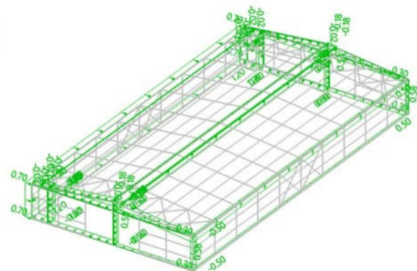
Slika 33.Vijetar1 - 0, + CPE, + CPI
