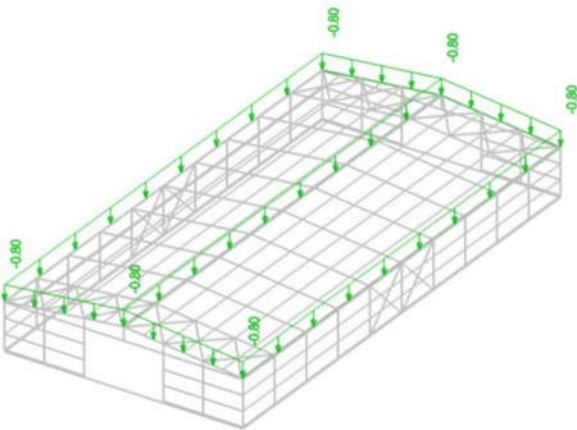
Slika 30.LC4 – snijeg
