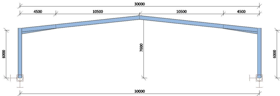
Slika 16. Upeti okvir
