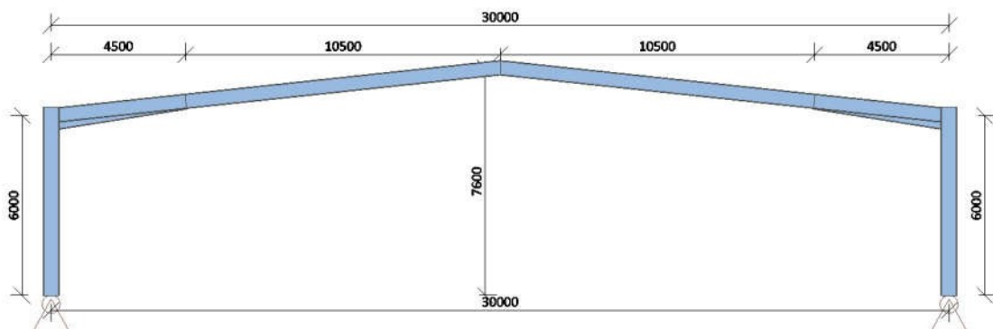
Slika 17. Dvozzglobni okvir
