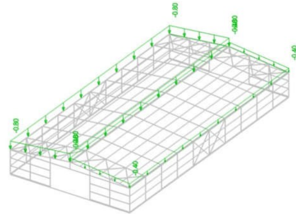
Slika 31.LC5 – snijeg lijeva stana krova
