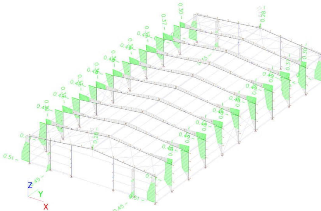
Slika 63. Iskoristivost elemenata (grede i stupa)
