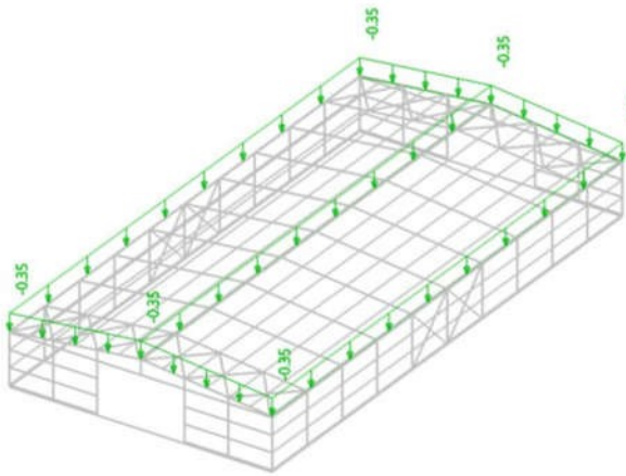
Slika 28.LC2 – dodatno stalno – krov
