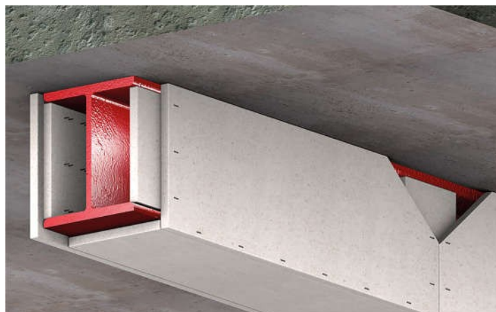
Slika 20. Protupožarne ploče [15]
