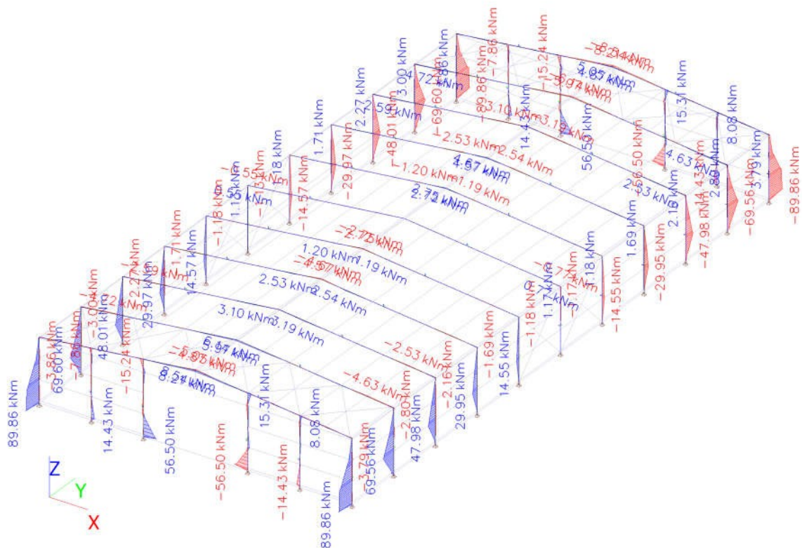
Slika 69. Rezne sile – Moment
